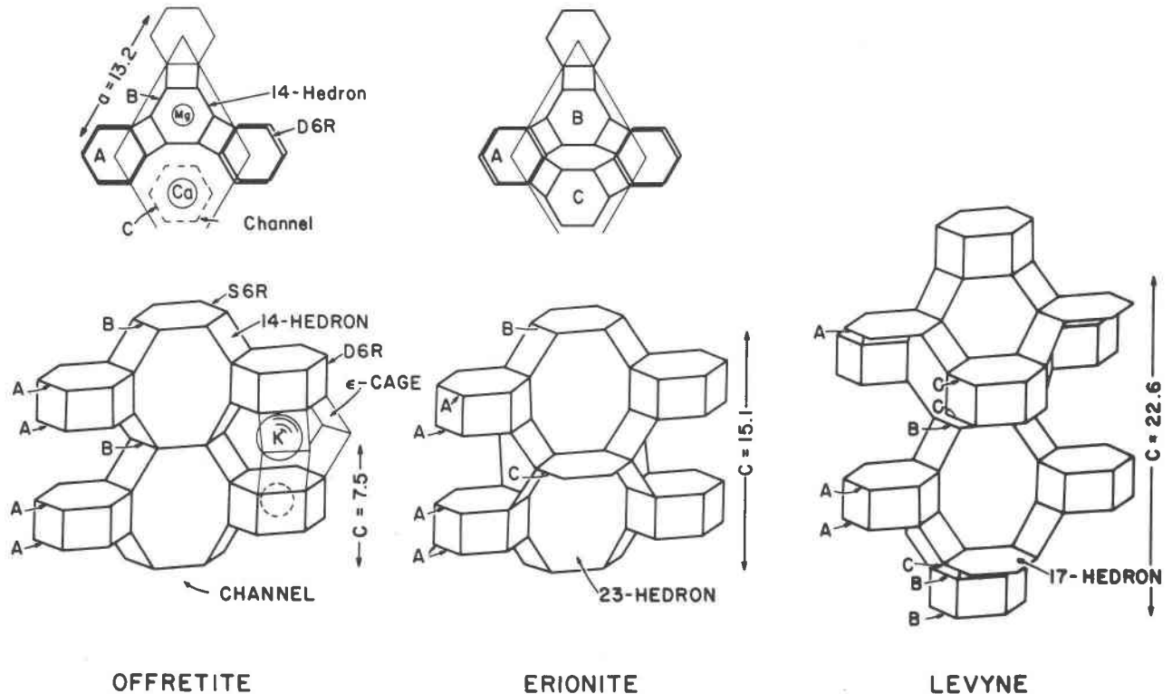
OFFRETITE
