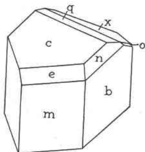
FIG. 2. Adularia.
