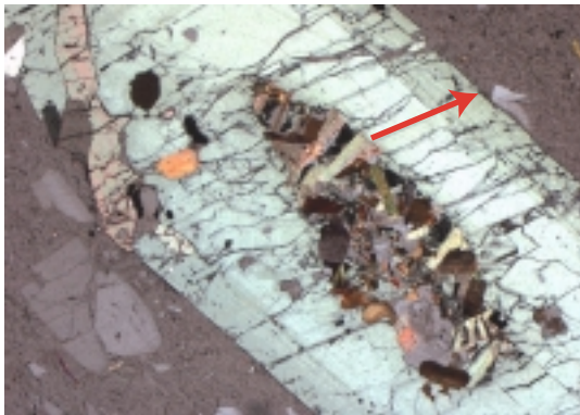
m) Pagosa Peak Dacite
